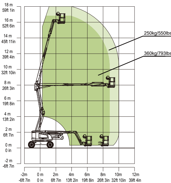
Диапазон движения ZA16J
